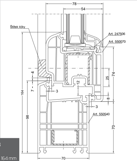
Rám BD 76 Křídlo Z 74 Skladebná výška 142 mm
