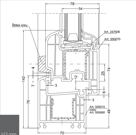
Rám BD 68 Křídlo Z 60 Skladebná výška 120 mm
