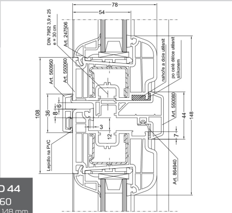
Rám BD 98 Křídlo Z 74 Skladebná výška 164 mm
