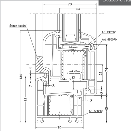
Rám BD 76 Křídlo Z 60 Skladebná výška 128 mm
