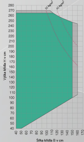
Křídlo s armováním 1358167 a REHAU vlepováním skel do křídlových ráhů, klapačka/velká klapačka s armováním
