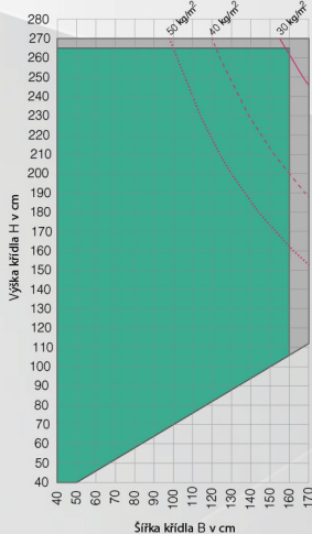
Křídlo s armováním 1358167 a REHAU vlepováním skel do křídlových ráhů
