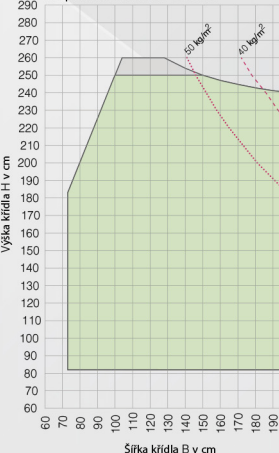
Křídlo s armováním 1358172, sloupek 92 s armováním 1358171
