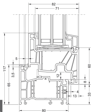
Rám 65 ARTEVO Křídlo 64 Odsazené křídlo ARTEVO Skladebná výška 117 mm
