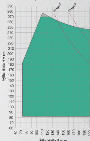
Křídlo s armováním 1358172, sloupek 92 s armováním 1358171, s REHAU vlepováním skel do křídlových ráhů
