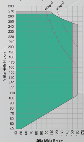
Křídlo s armováním 1358167 a REHAU vlepováním skel do křídlových ráhů, klapačka/velká klapačka s armováním
