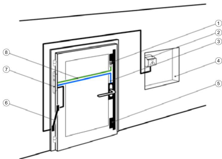
Obr. 1: Přehled systému
